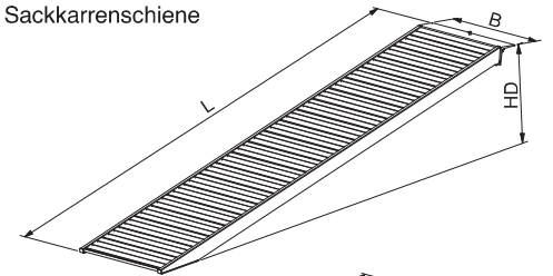
Sackkarrenschiene faltbar
